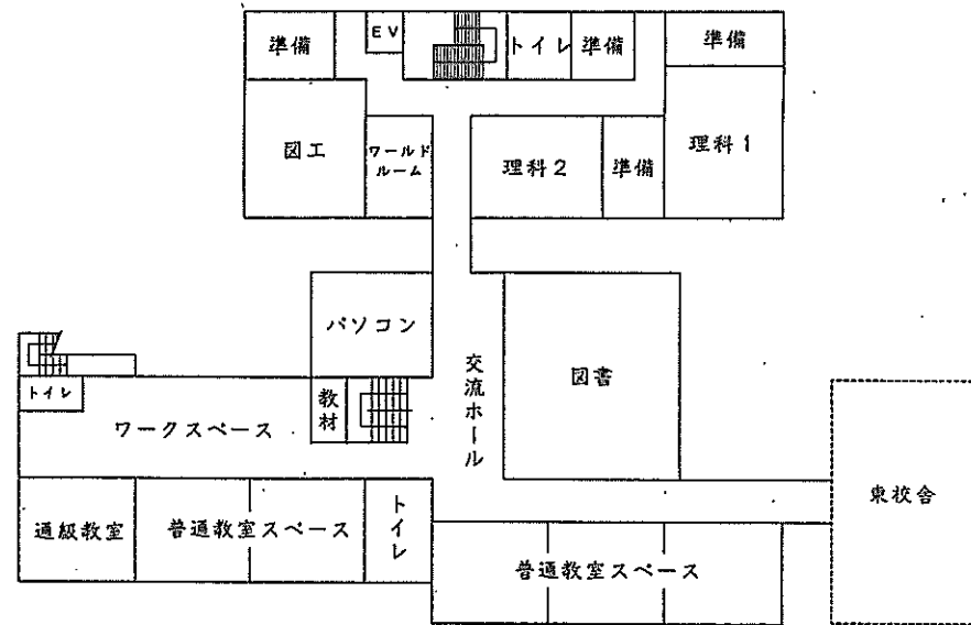
2階平面図
