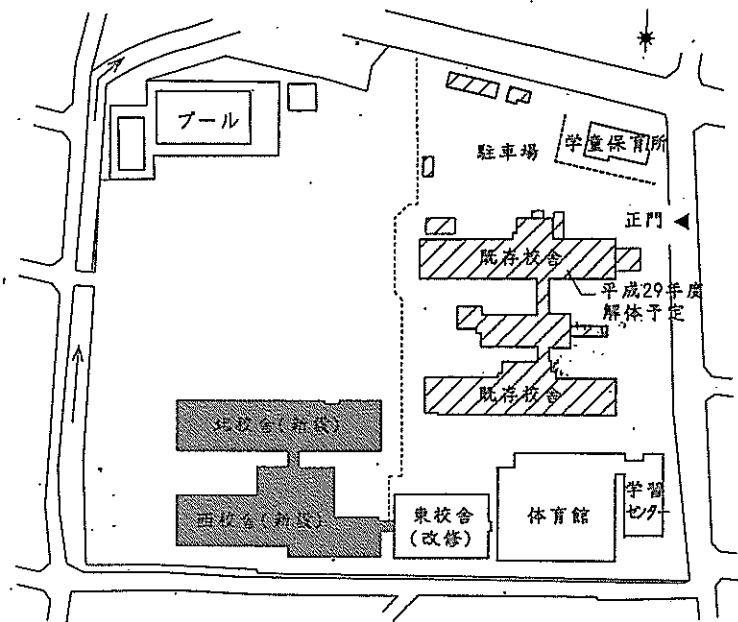
配置図
