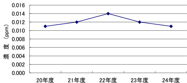
窒素酸化物(NOx)の経年変化 (大東支所)
