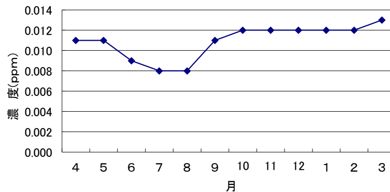
H24年度窒素酸化物(NOx)の月別変化(大東支所)
