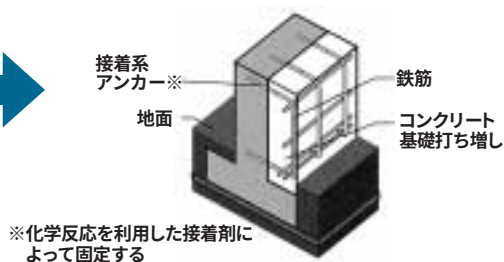
鉄筋コンクリート基礎の打ち増し
