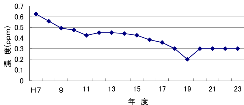
一酸化炭素(CO)の経年変化(自排局)
