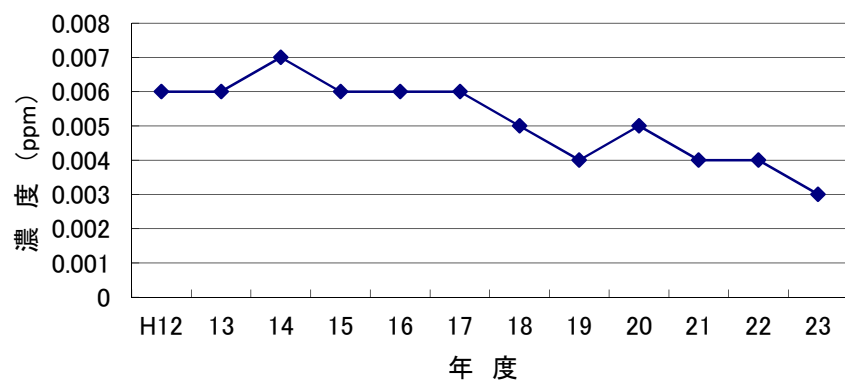
一酸化窒素(NO)の経年変化 (大東支所)
