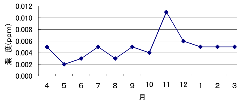
H23年度一酸化窒素(NO)の月別変化(市役所)
