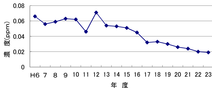
窒素酸化物(NOx)の経年変化(自排局)
