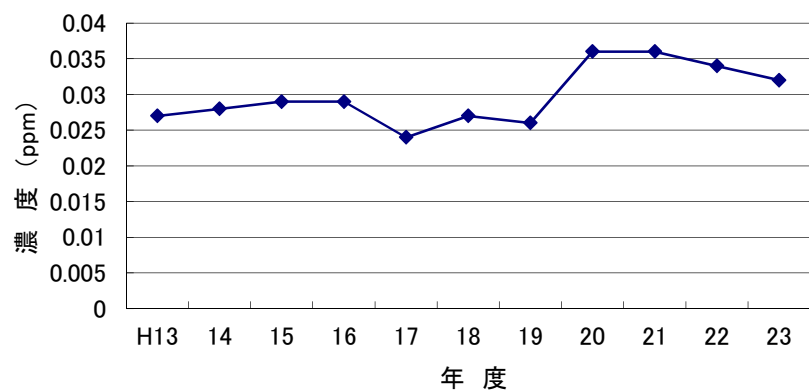
オキシダント(Ox・24h)の経年変化 (大東支所)
