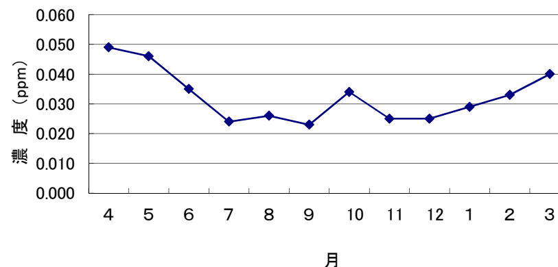
H23年度 オキシダント(Ox・24h)の月別変化 (大東支所)
