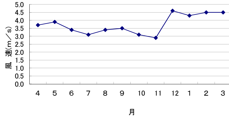
H23年度 WS(風速)の月別変化(市役所)
