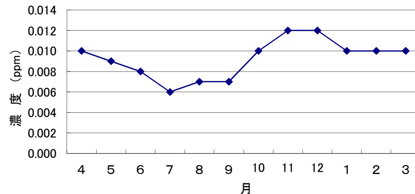
H23年度 二酸化窒素(NO2)の月別変化 (大東支所)
