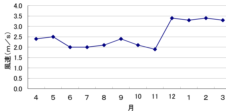
H23年度 風速(WS)の月別変化(自排局)
