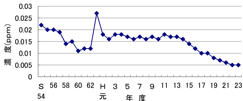
一酸化窒素(NO)の経年変化(市役所)
