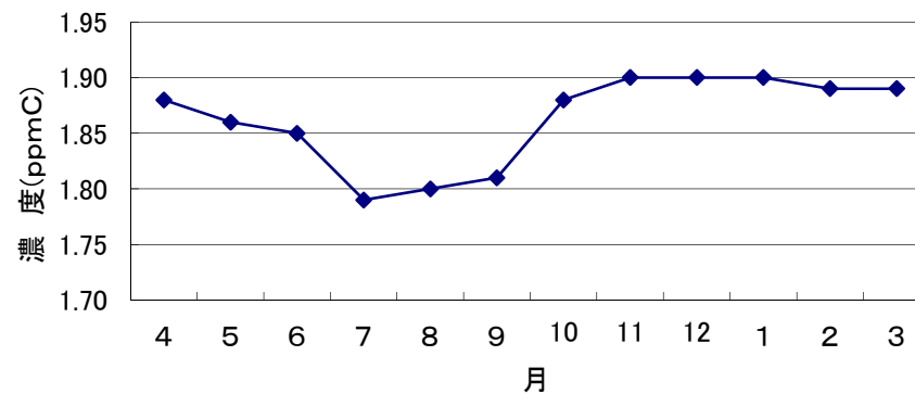
H23年度 炭化水素(HC)の月別変化
