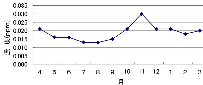
H23年度 窒素酸化物(NOx)の月別変化(自局)
