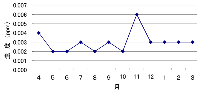
H23年度一酸化窒素(NO)の月別変化(大東支所)
