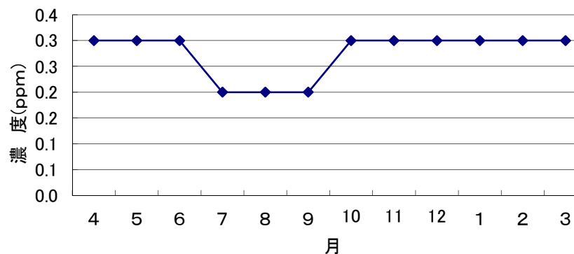
H23年度 一酸化炭素(CO)の月別変化(自排局)
