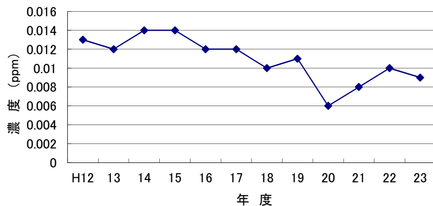
二酸化窒素(NO2)の経年変化 (大東支所)
