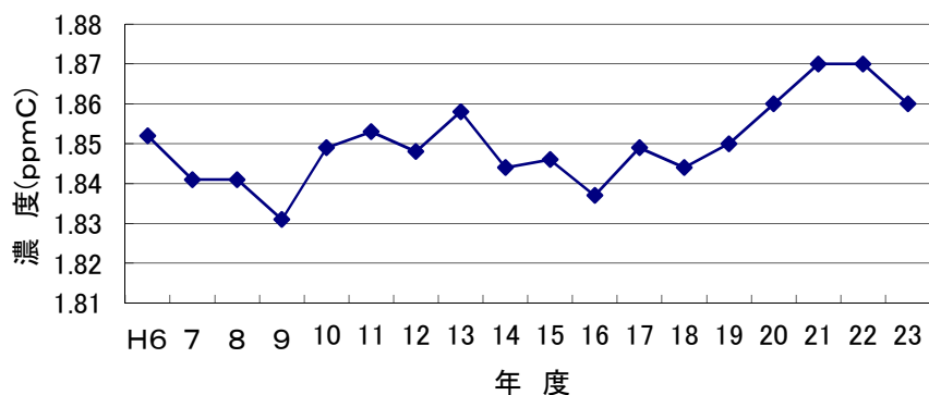
炭化水素(HC)の経年変化(自排局)
