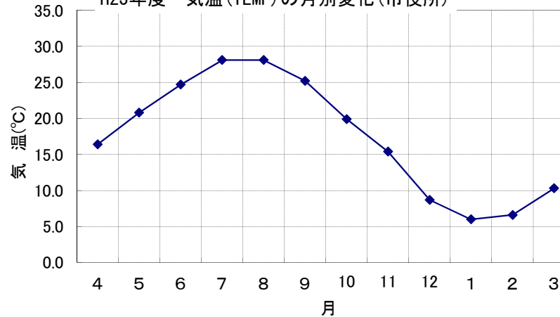
H23年度 気温（TEMP）の月別変化（市役所）
