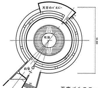
天空バルコニー平面図 S=1:300
