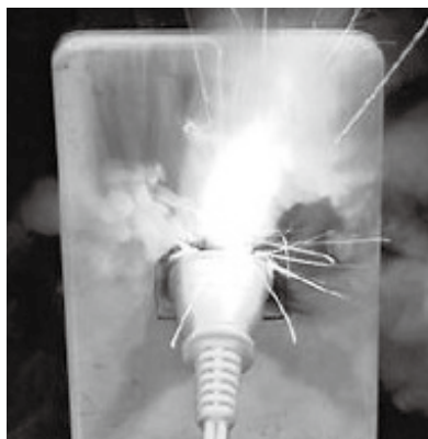
【NITEの再現実験】 トラッキング現象による発火
